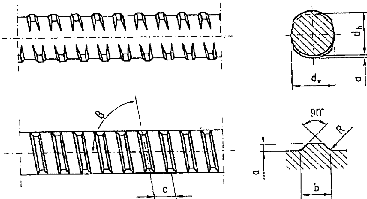
Gewinderippe
