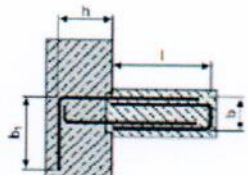
Typ KHS Konsolentyp für weit ausragende Konsolen
