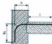
Typ BA Biegesteifer Anschluss
