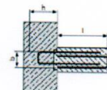
Typ KS Konsolentyp für weit ausragende Konsolen
