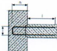
Typ S1 Steckbügel in einem Blech
