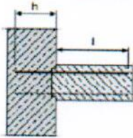
Typ W (Typ W 2reihig) Einfacher Winkel
