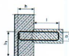
Typ BK 1) Konsole, Bügel geschlossen
