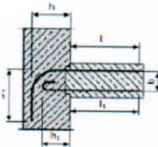
Typ BA mit Druckstab Biegesteifer Anschluss
