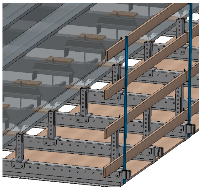
Stütze
