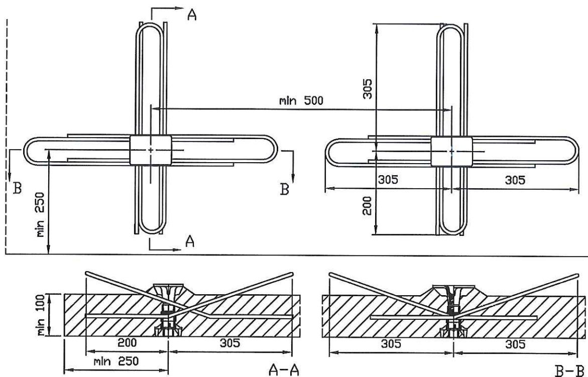
Bild 15: Einbau in Fertigteilen (hier: Bauzustand ohne Ortbeton)
