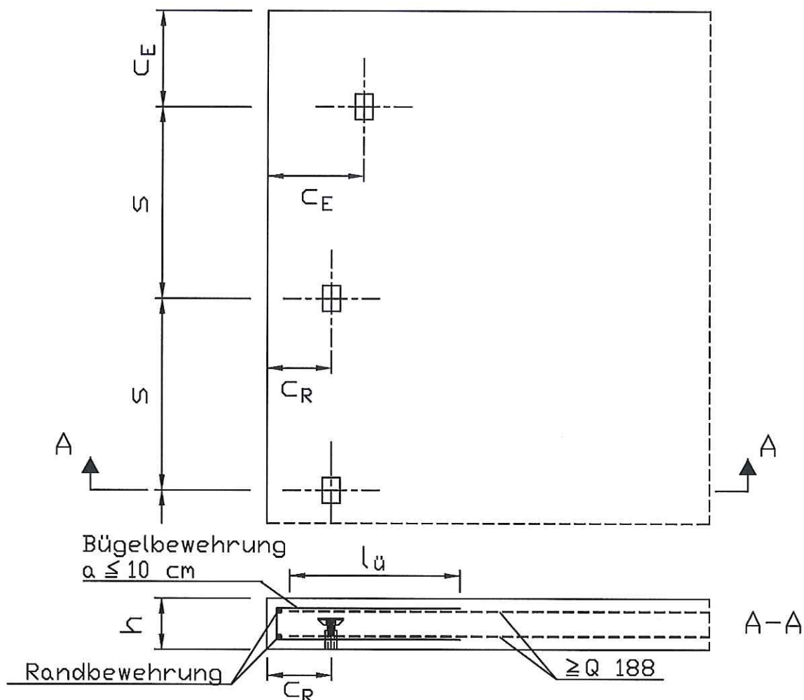
Bild 13: (Mindest-) Abstände, Zusatzbewehrung
