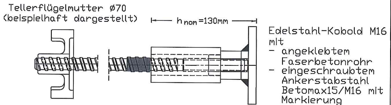
Bild 11: Einzelteile im montierten Zustand
