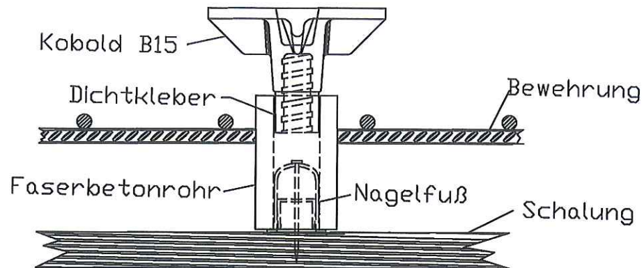
Bild 3: Montage auf der Schalung
