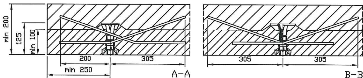
Bild 16: Einbau in Fertigteilen (hier: Bauzustand mit Ortbeton)
