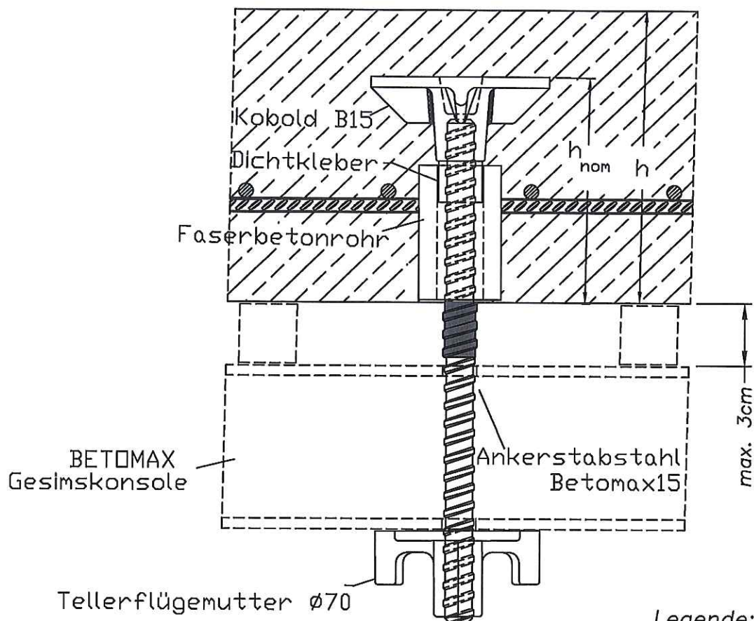
Bild 3: Montage auf der Schalung
