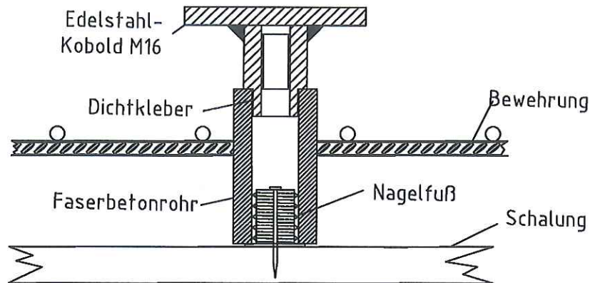
Bild 5: Montage auf der Schalung
