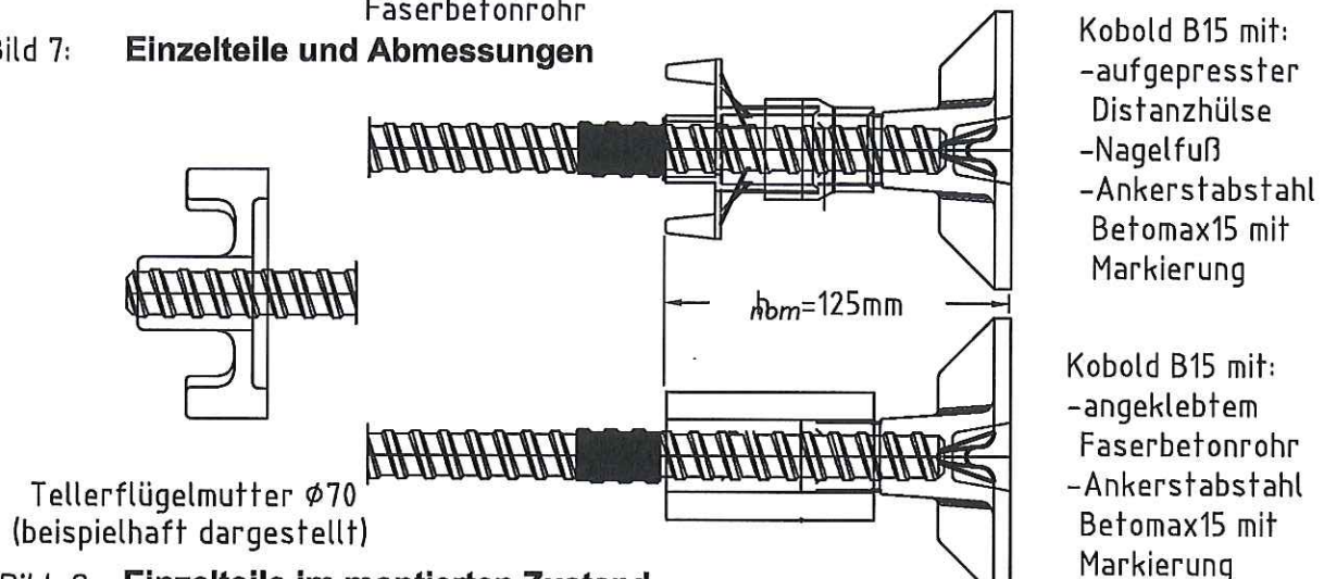
Bild 8: Einzelteile im montierten Zustand
