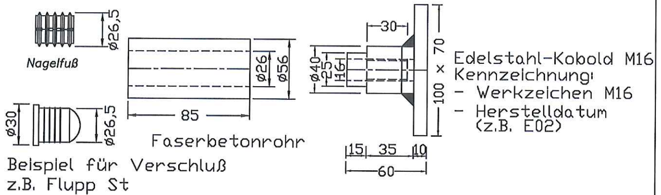
Bild 10: Einzelteile und Abmessungen
