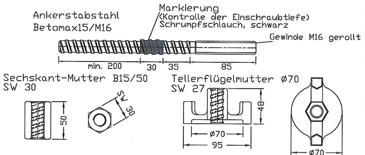
Bild 12: Ankerstabstahl, Sechskant- und Tellerflügelmutter
