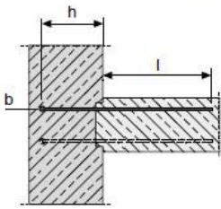
Typ WH Winkel mit Haken in Blechrichtung
