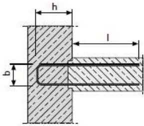
Typ S1 Steckbügel in einem Blech
