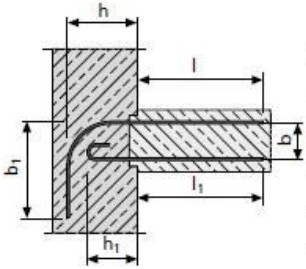
Typ BA mit Druck- stab – Biegesteifer Anschluss
