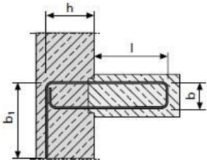
Typ BK Konsole Bügel geschlossen
