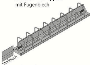
COMAX® WU Typ S1 mit Fugenblech
