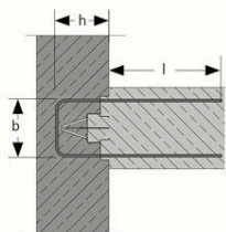
COMAX® WU Typ S1 mit Fugenblech
